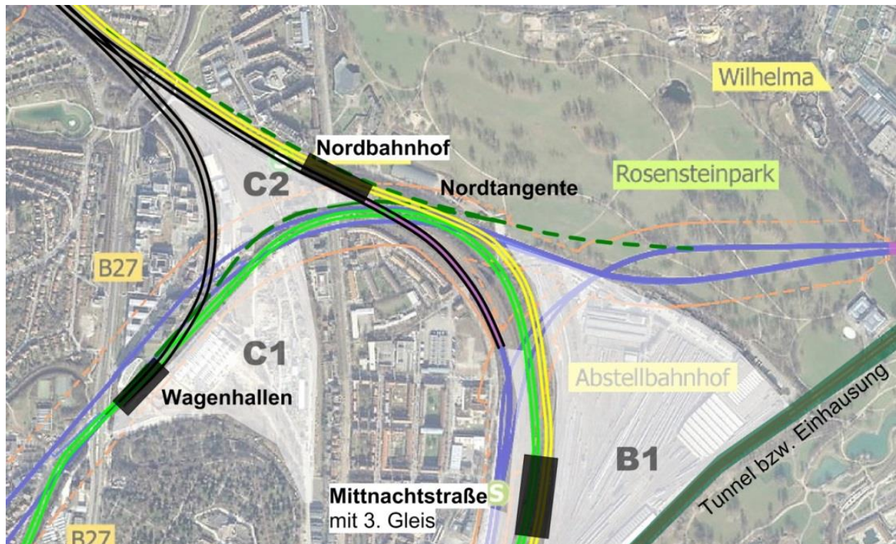
Abbildung 8: VCD-Vorschlag zum Nordkreuz
