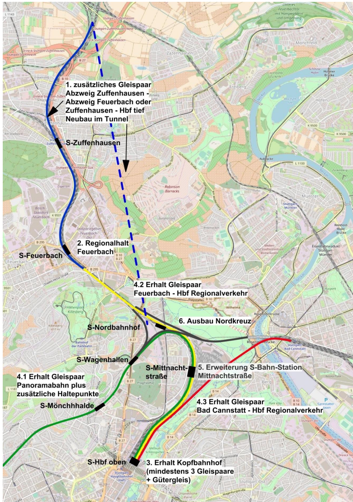
Abbildung 3: Vorschläge des VCD zum Ausbau der Schieneninfrastruktur
