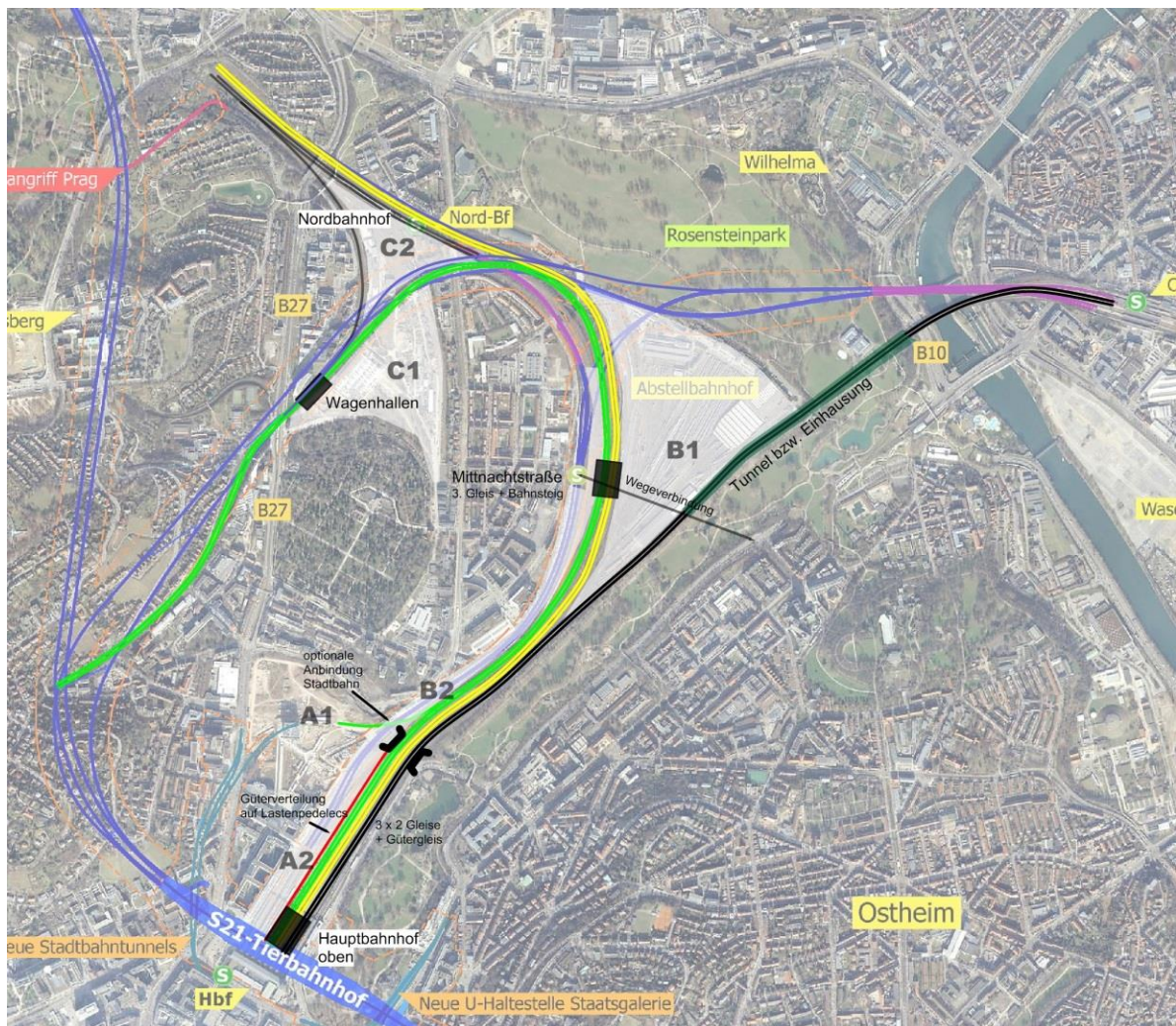
Abbildung 11: Flächenbedarf des VCD-Vorschlags im Rosensteinviertel
