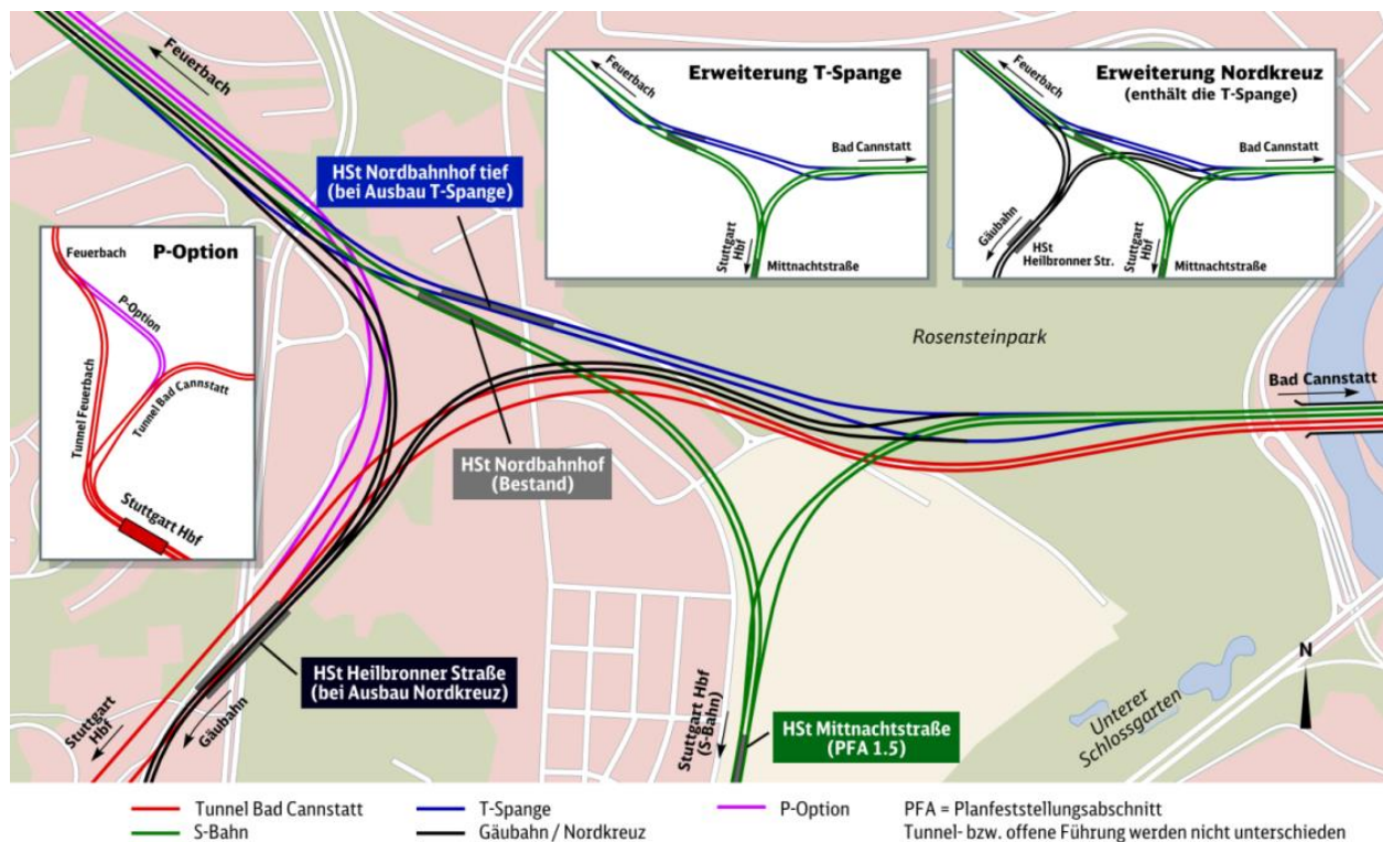
Abbildung 7: Planungsvarianten zum Nordkreuz bei Stuttgart 21
